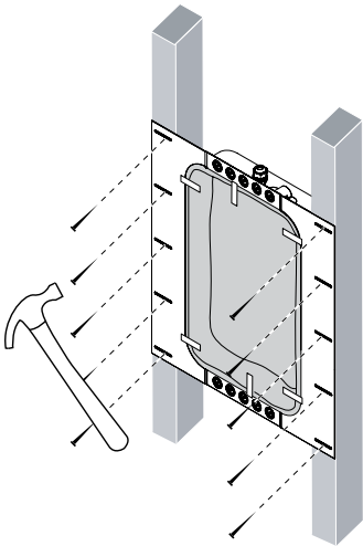
图10 背箱板墙筋(托梁)安装
