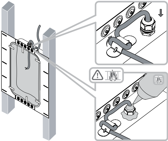
图11 接线安装
