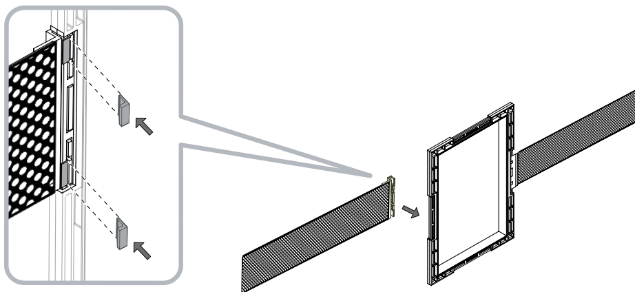
6. ábra A pántok rögzítése
