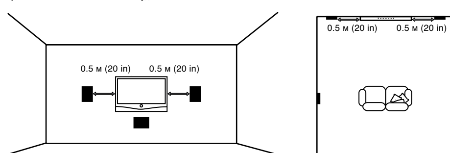
Рисунок 2 Размещение AC
