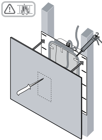
图12 石膏板(石膏灰泥板)安装
