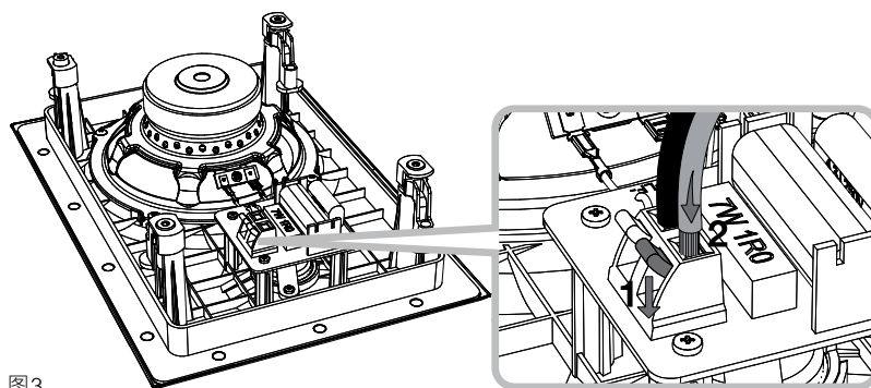
图3 接线连接
