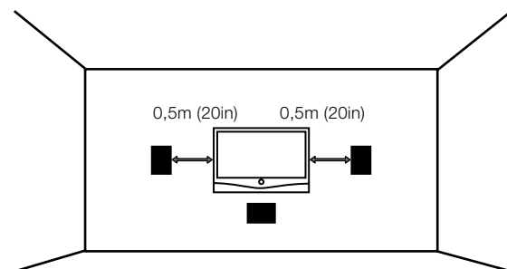
Obrázek 2 Umístění
